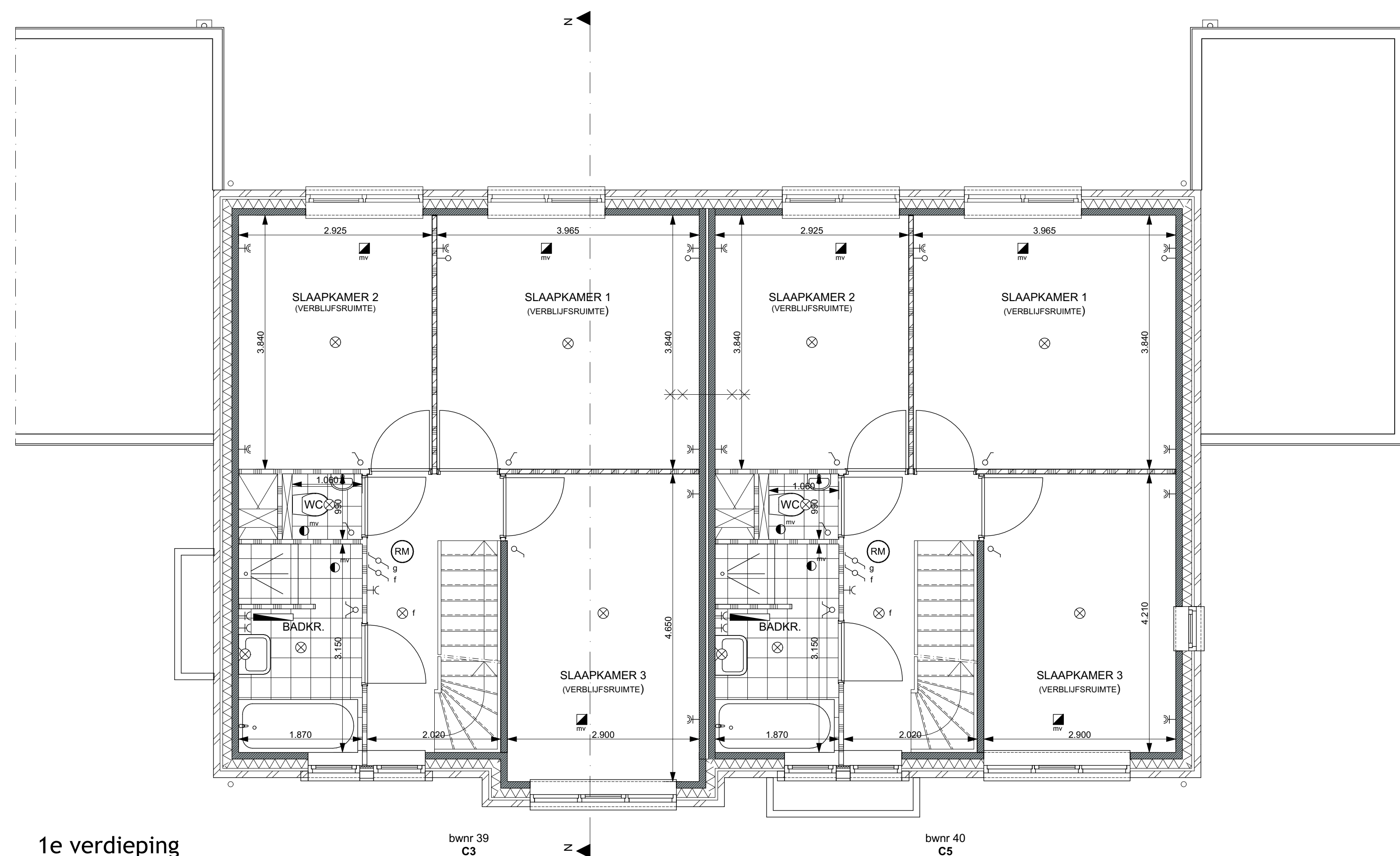
1e verdieping
