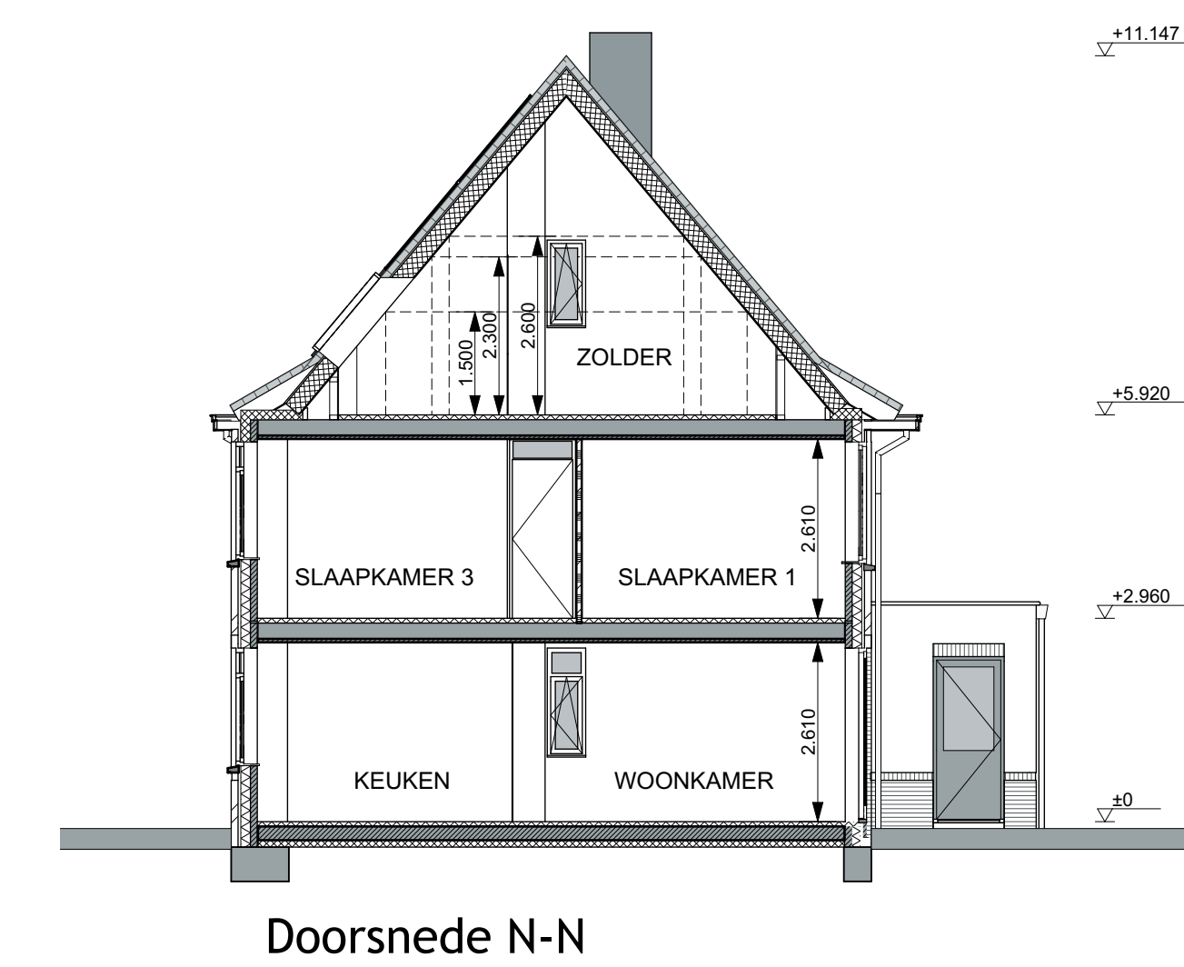
Doorsnede N-N
