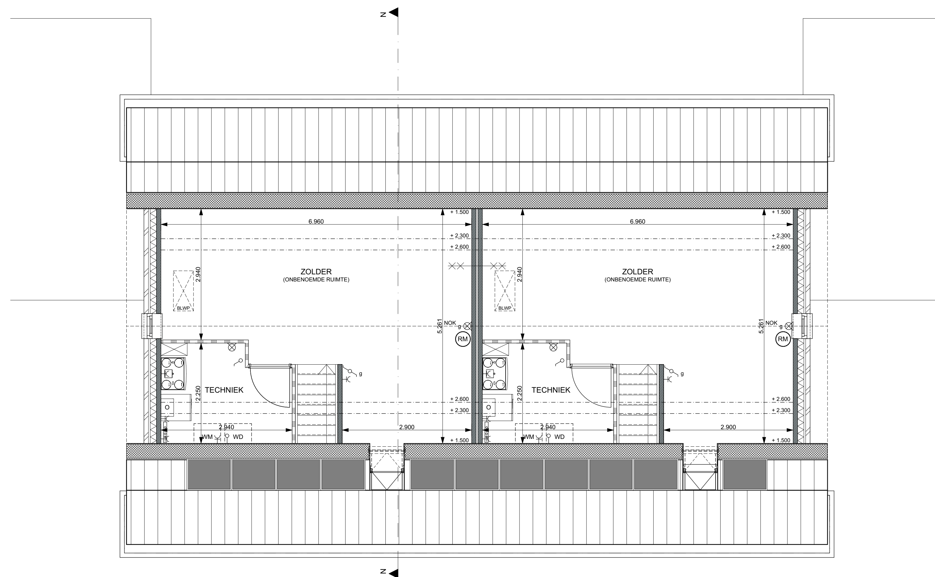
2e verdieping
